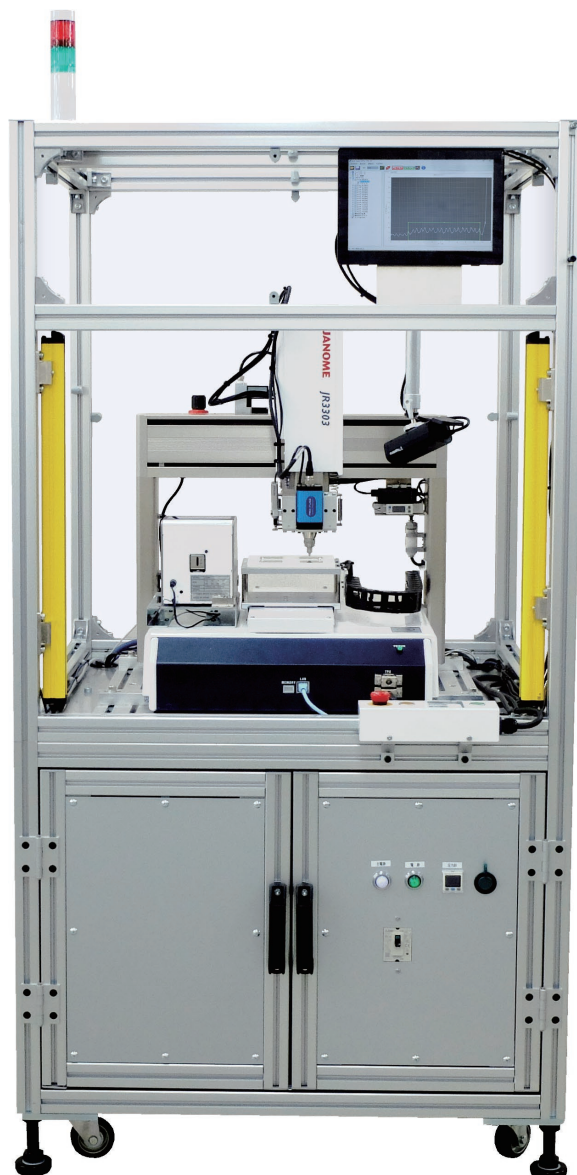
ねじ締めロボット自動化設備例※
